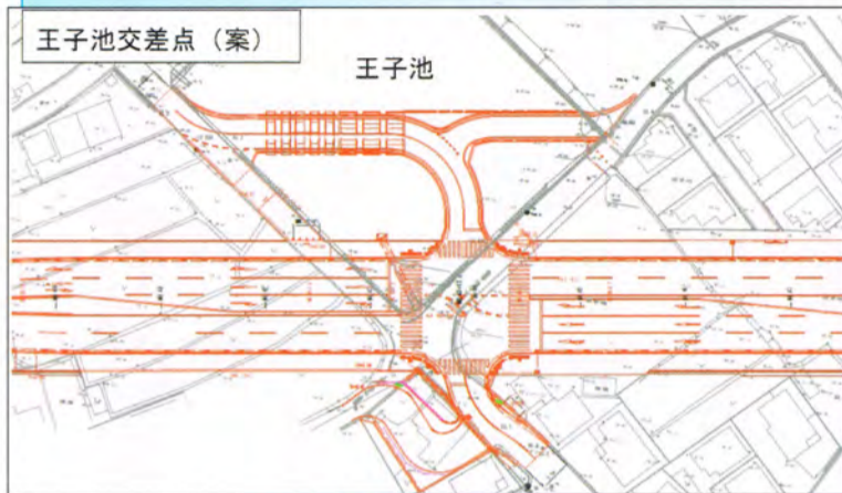
王子池交差点の設計案
